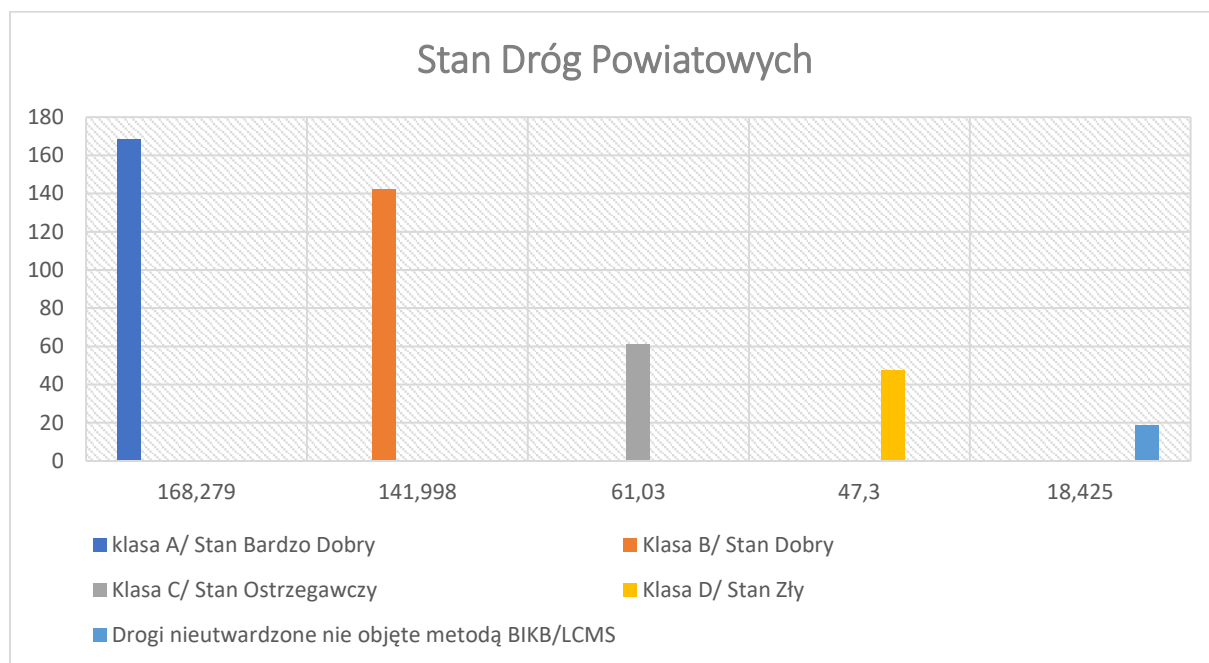
Rys. 3. Stan dróg powiatowych
